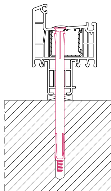
Дюбель
