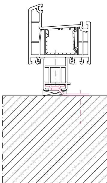
Монтажная (анкерная) пластина
