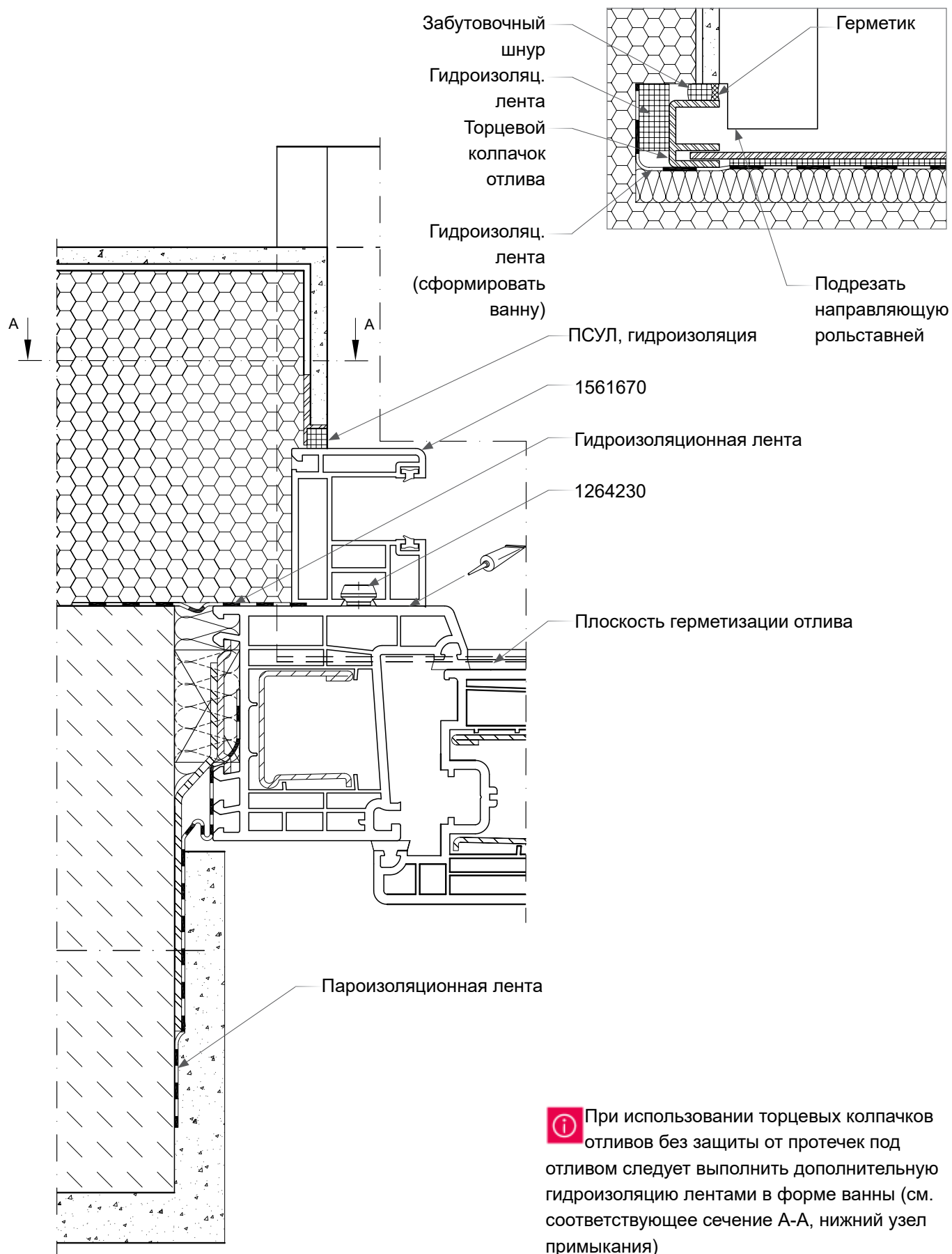
Сечение А-А:
