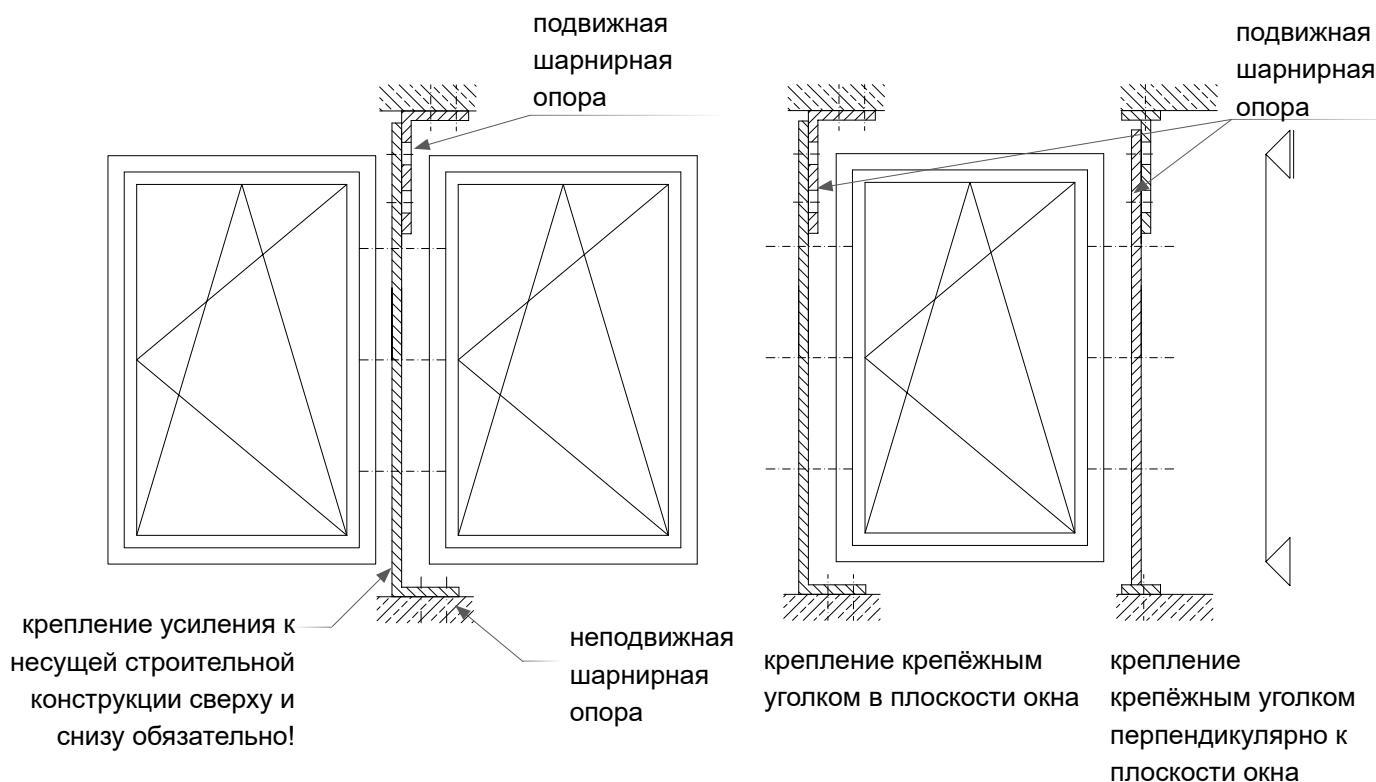
Рис. 16: Соединения оконных блоков
