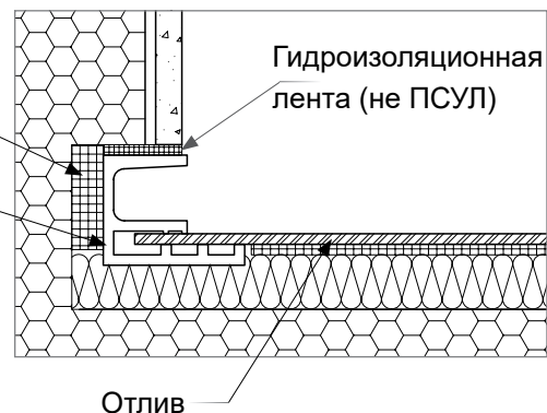
Сечение А-А:
