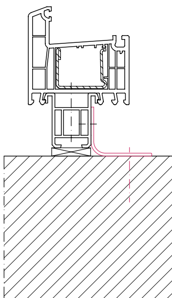
Уголок
