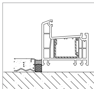
обмазочная гидроизоляция между коробкой и штукатурным слоем
