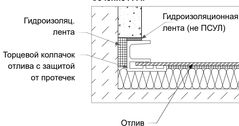
Сечение А-А:
