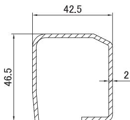
3728 🌐 Армирование 46.5 * 42.5 мм
