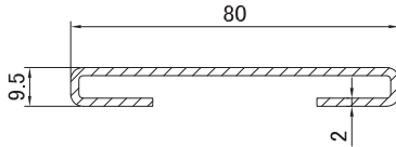
1712 Армирование 9.5 * 80.0 * 2.0 мм
