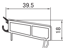
3136 Штапик 39.5 мм
