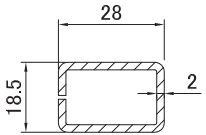
1703 Армирование 18.5 * 28.0 мм
