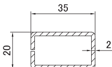
1707 Армирование 20.0 * 35.0 мм
