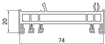
2315 Расширитель 20 мм
