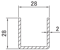
1700 Армирование 28.0 * 28.0 мм
