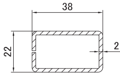
1720 Армирование 22.0 * 38.0 мм
