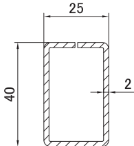
3716 Армирование 40.0 * 25.0 мм
