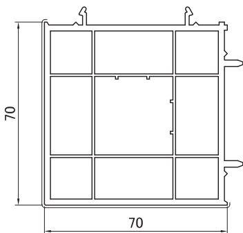
1243 Соединительный профиль 90°
