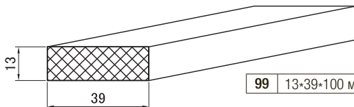
1339 🌐 Компенсационная вставка
