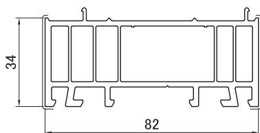
2220 Расширитель 34 мм
