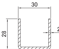
1704 Армирование 28.0 * 30.0 мм
