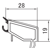
1124 Штапик 28.0 мм
