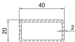
2724 Армирование 20.0 * 40.0 мм
