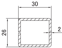
3709 Армирование 26.0 * 30.0 мм
