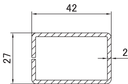
3713 Армирование 27.0 * 42.0 мм
