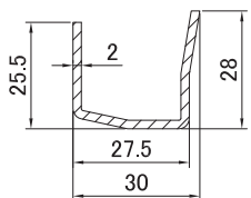
3764 🌐 Армирование 25.5 * 27.5 * 28.0 мм
