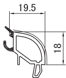
1132 Штапик 19.5 мм
