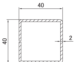
3797 🌐 Армирование 40.0 * 40.0 мм
