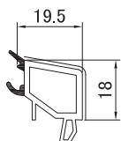
3116 Штапик 19.5 мм
