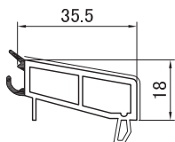
3132 Штапик 35.5 мм
