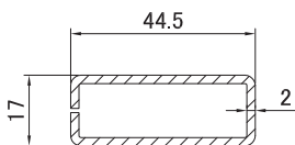
1724 Армирование 17.0 * 44.5 мм
