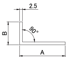
71***** Уголок 90°
