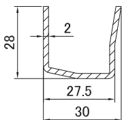
3720 Армирование 28.0 * 30.0 мм
