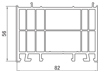
2221 Расширитель 56 мм
