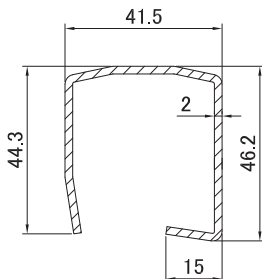
1710 Армирование 44.3 * 41.5 * 46.0 * 2.0 мм
