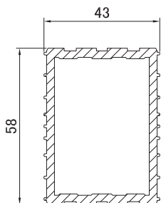
3732 🌐 Армирование 58.0 * 43.0 мм
