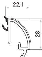
2240 Штапик 22.0 мм
