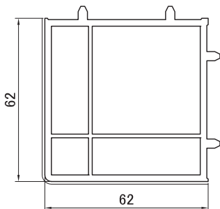
3295 Соединительный профиль 90°
