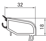
7124 Штапик 32.0 мм
