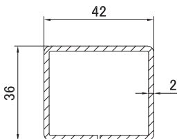
3727 Армирование 36.0 * 42.0 мм
