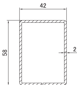
3736 🌐 Армирование 58.0 * 42.0 мм
