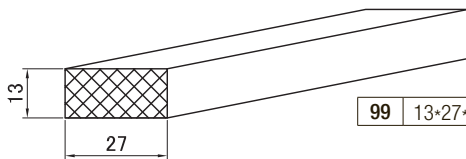
1327 🌐 Компенсационная вставка
